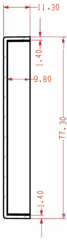
SECTION A-A
